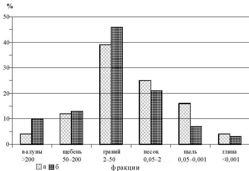
Рис. 1.8. Осредненный гранулометрический состав селеформирующих грунтов (а) и селевых отложений (б). Крымские горы, Украина (по А. С. Тищенко, 1992)
