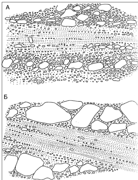
Рис. 1.10. Строение отложений селевого паводка («сухой» реки) на р. Апахончич, подножье Ключевой сопки, Камчатка. Отложения валунно-галечно-песчаные, слоистость параллельнолинейная. (И. В. Мелекесцев и др., 1970)
