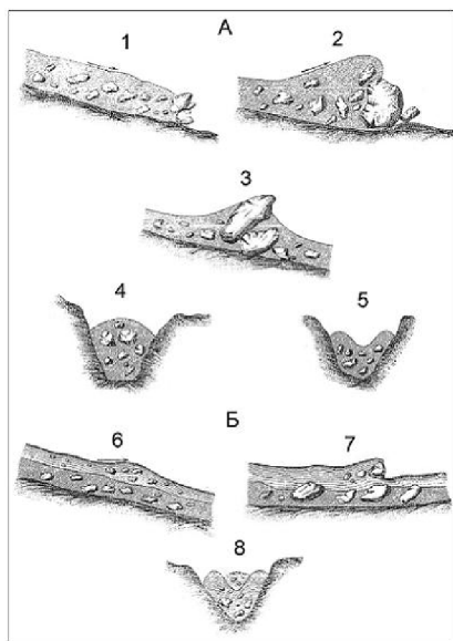
Рис. 1.3. Изменения состава и форм движения селя в процессе его схода. А – селевой грязекаменный поток: 1 – сель с глыбами в передней части фронта; 2 – реакция фронта потока на препятствие; 3 – воздымание глыб над поверхностью потока; 4 – форма поверхности селя при подъеме уровня; 5 – форма поверхности селя при спаде уровня. Б – слой воды на поверхности грязекаменного селя: 6 – в продольном разрезе; 7 – слой воды включает крупные обломки; 8 – расположение слоя воды в поперечном разрезе (по П. Демонце, 1891)
