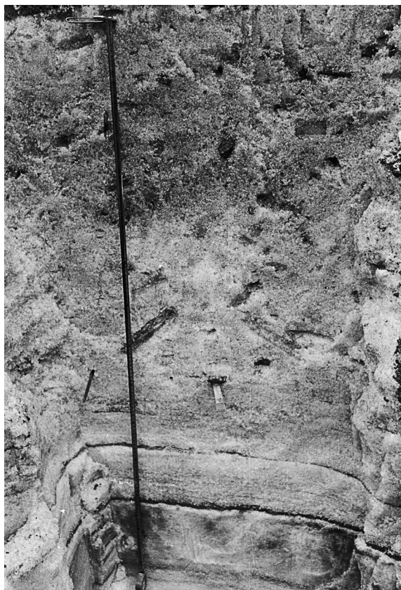
Рис. 1.14. Строение отложений водоснежного потока: бесструктурная масса снега, насыщенного мелкоземом и щебнем; у подошвы разреза – слои руслового снежника. Бассейн р. Вуоннемйоок, Хибины, 1977 г.
