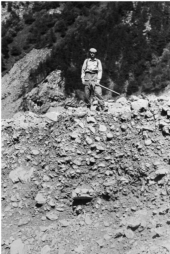
Рис. 2.2. Состав отложений грязекаменного селя на конусе выноса р. Касайкомдон, Сев. Кавказ, 1986 г.
