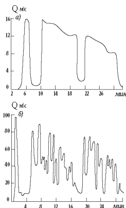
Рис. 1.4. Гидрограф водного пуща в Чемолганский очаг (а) и соответствующий ему гидрограф селевого потока (б) в эксперименте 1973 г. (Б. С. Степанов, Т. С. Степанова, 1991)
