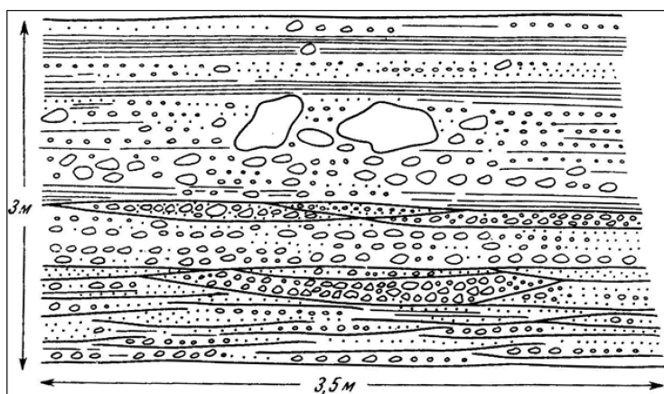
Рис. 1.10. Строение отложений селевого паводка («сухой» реки) на р. Апахончич, подножье Ключевой сопки, Камчатка. Отложения валунно-галечно-песчаные, слоистость параллельнолинейная. (И. В. Мелекесцев и др., 1970)
