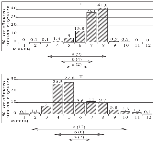
Рис. 1.11. Распределение случаев схода селей за год на Сев. Кавказе (I) и в Копетдаге (II). Периоды: а – селеопасный; б – основной селеопасный; в – наибольшей селевой опасности
